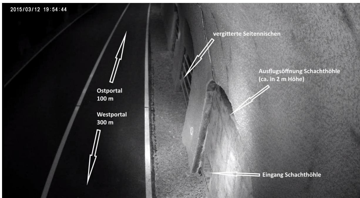
Abbildung 3: Kameraansicht der Ausflugsöffnung der Schachthöhle in der Tunnelröhre
