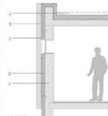
Fassadenschnitt M 1:25
